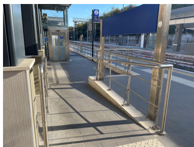
Fig.5 rampe di accesso all'ascensore sul binario 1 della stazione Roma San Pietro
